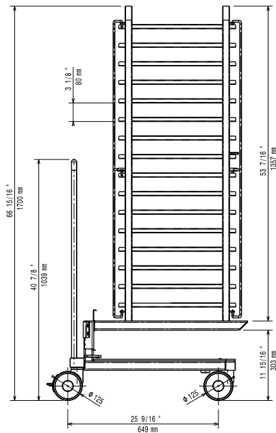
Front aanzicht
